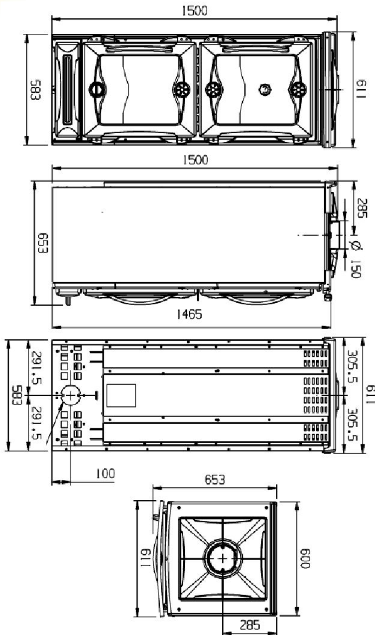
Kaminofenherd mit optionaler Grillfunktion und grosser Panoramasscheibe
