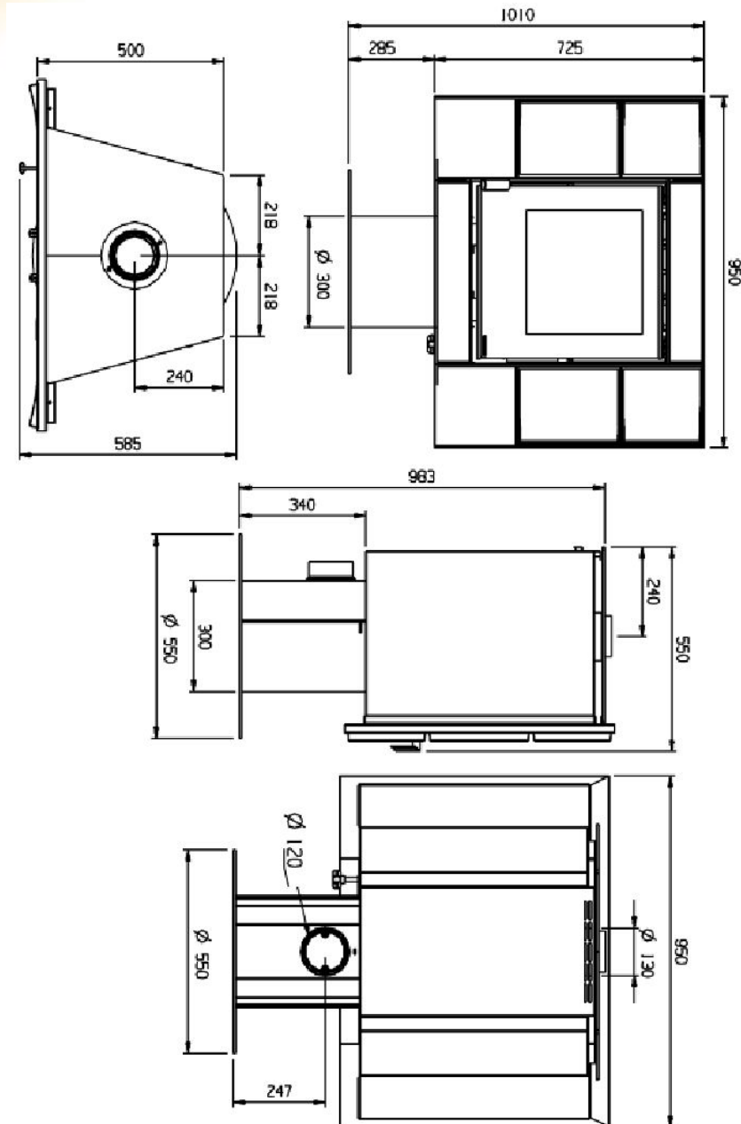
Drehbarer Ofen mit großer Brennkammer
